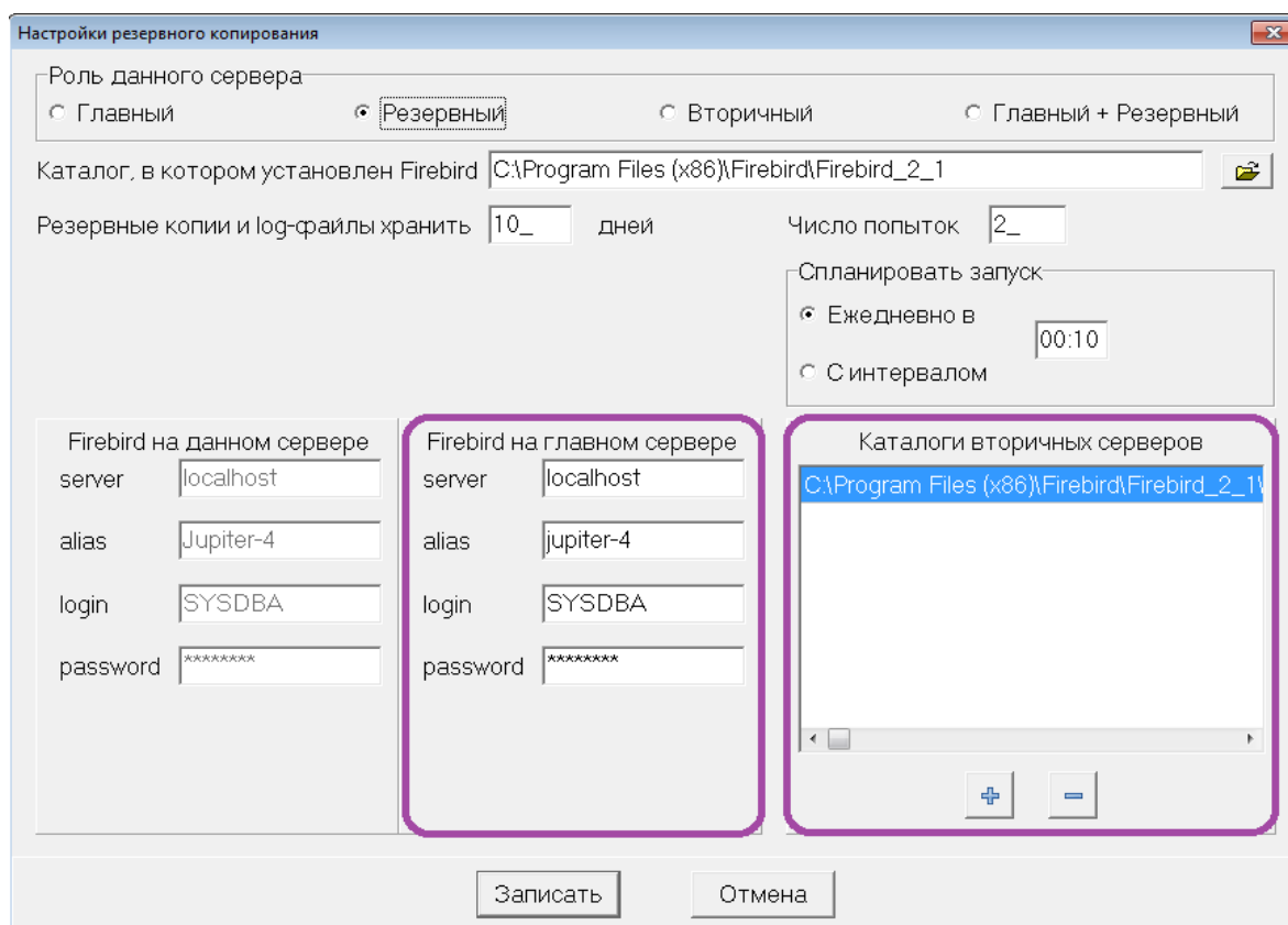
Рисунок 5.4. Настройка параметров работы в режиме «Резервный»
