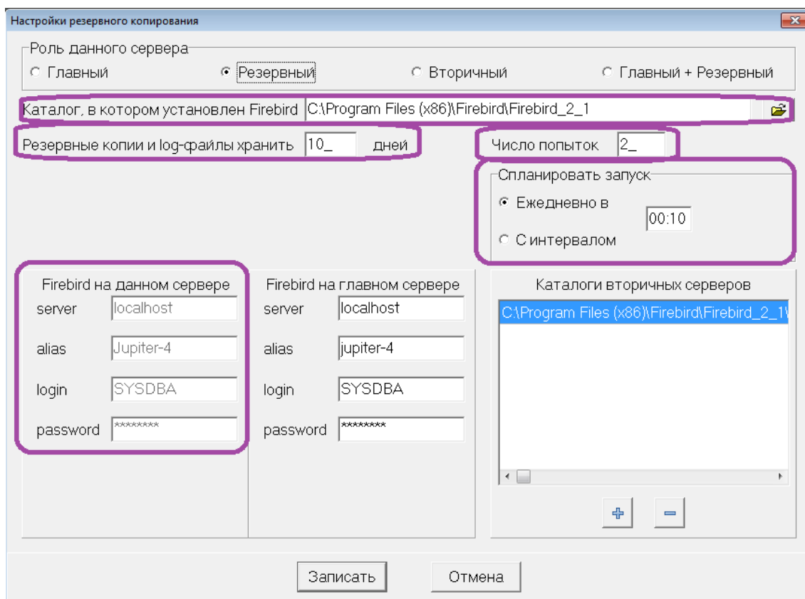
Рисунок 5.3: Обязательные параметры выполнения резервного копирования
