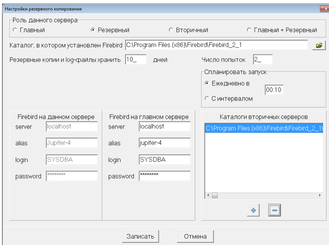
Рисунок 5.2. Задание параметров выполнения резервного копирования
