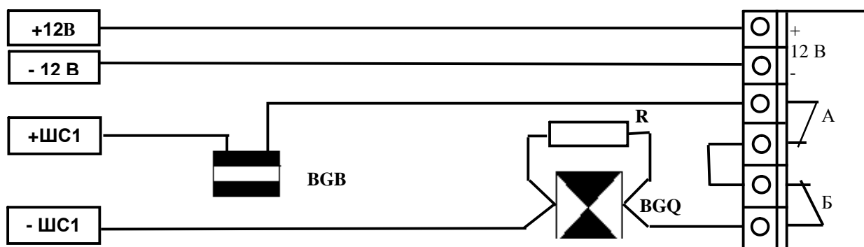
Рис.2. Пример шлейфа охранной сигнализации
